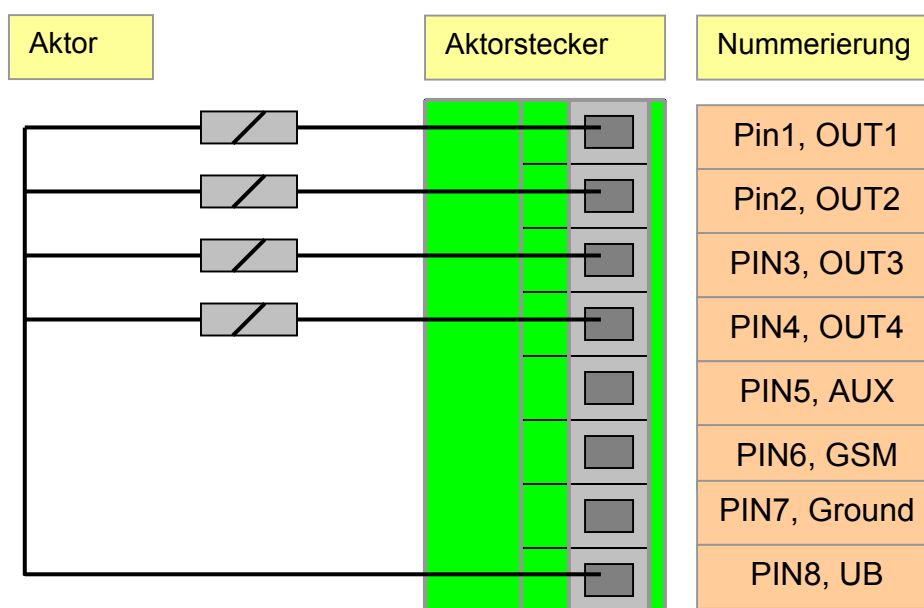
Bild 13: Beschaltung der Aktor-Ausgänge mit Relais
